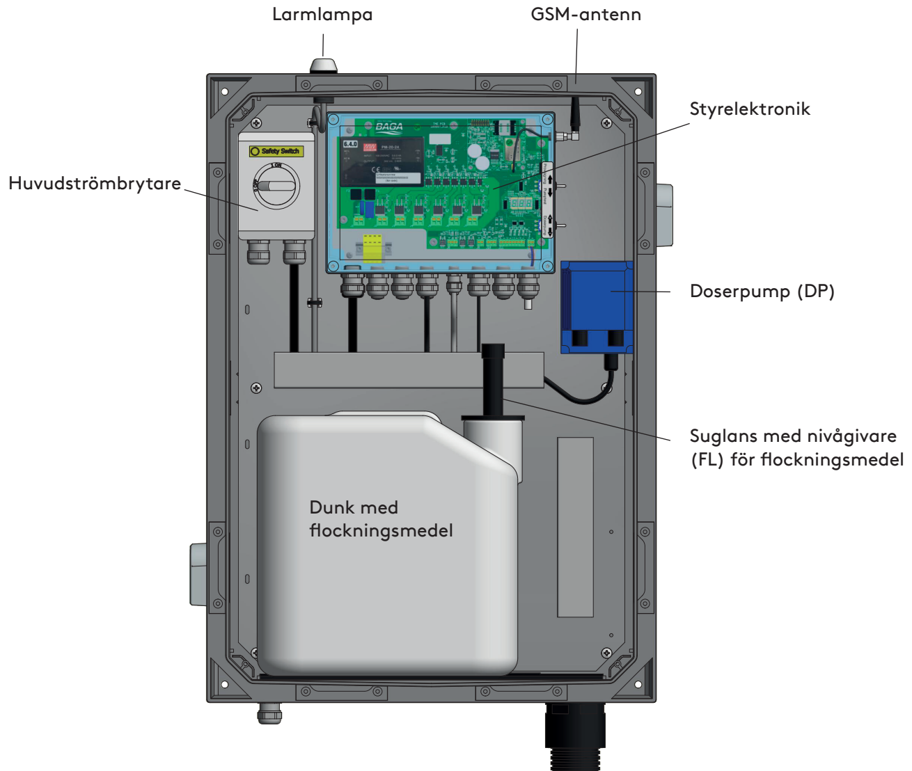
Figur 2. Översikt Automatikskåp
